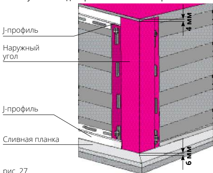
Схема установки доборных элементов и вертикального сайдинга
