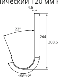
Кронштейн желоба металлический 120 мм Классика
