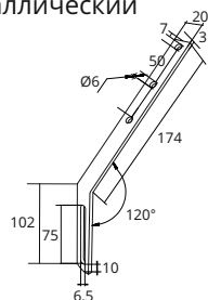
Удлинитель кронштейна желоба металлический
