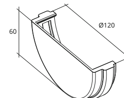
Заглушка желоба ПВХ 120/90
