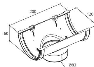
Воронка ПВХ 120/90
