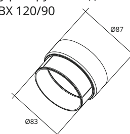
Хомут трубы ПВХ 120/90
