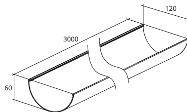
Желоб ПВХ 120/90 3м
