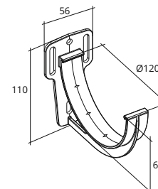
Кронштейн желоба ПВХ 120/90
