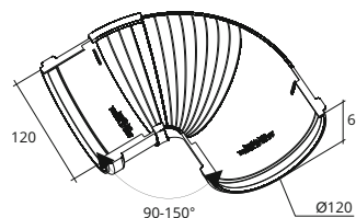
Угол желоба 90°-150° ПВХ 120/90
