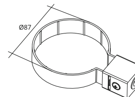
Хомут трубы Kликер ПВХ Premium 120/90
