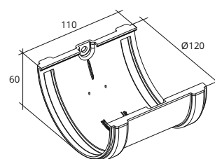
Соединитель желоба ПВХ 120/90
